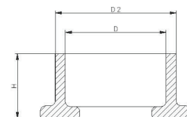
Demontagewerkzeug disassembling tool
